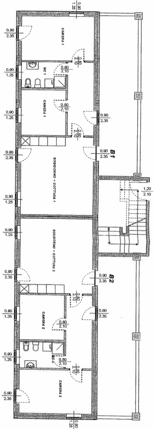
EDIFICIO B . PIANTA PIANO TERRA
